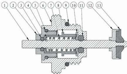
Конструкция и спецификация материалов балансировочного клапана
