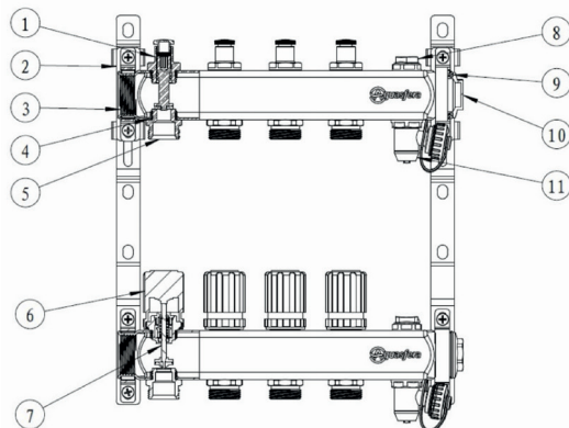
Конструкция и спецификация материалов коллекторной группы
