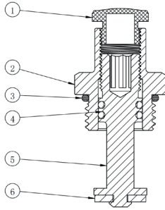
Конструкция и спецификация материалов балансировочного клапана коллектора 9502
