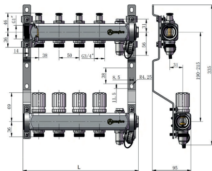
Габаритные и присоединительные размеры коллекторных групп 9502 Aquasfera
