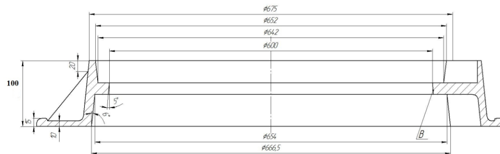
Люк чугунный круглого дождеприемника типа ДБ2 (В125) 1-60 ГОСТ 3634 - 2019.
